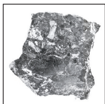
Breccia
