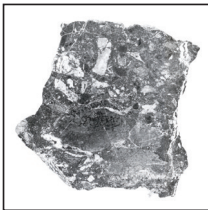
Breccia
